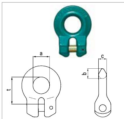
Gabelverbinder Eye-Connector
