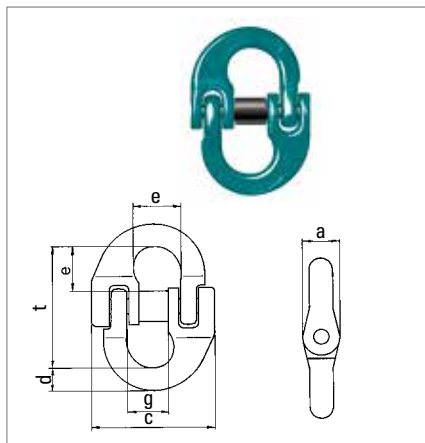
Bügeschloss Coupling
