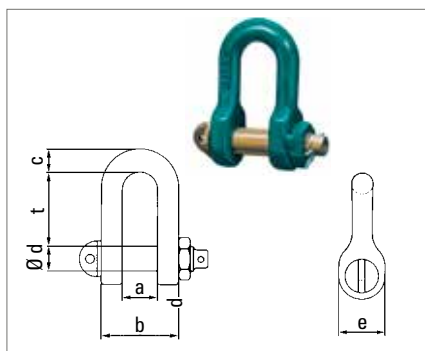
Verbindungsschäkel Shackle
