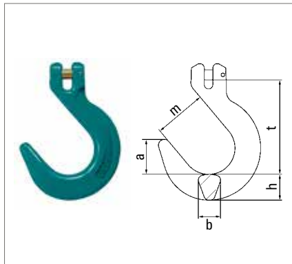
Weitmaulhaken Foundry hooks
