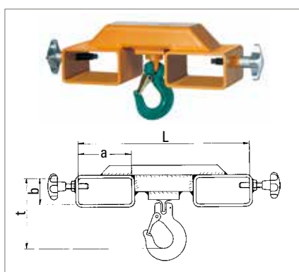
Aufsteckschuh für Gabelstapler - doppelt -
