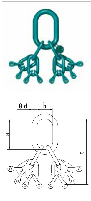
Sonderaufhängekopf
