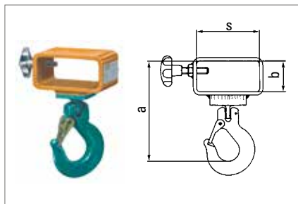
Aufsteckschuh für Gabelstapler
